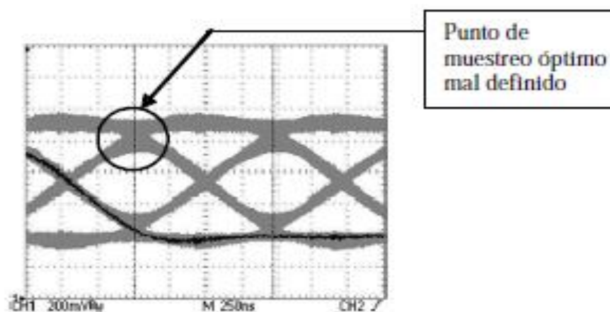
Figura 12-4. Diagrama en ojo con distorsión
